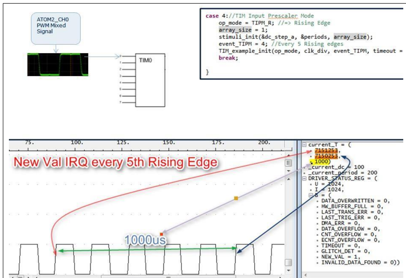
图16 TIPM示例
