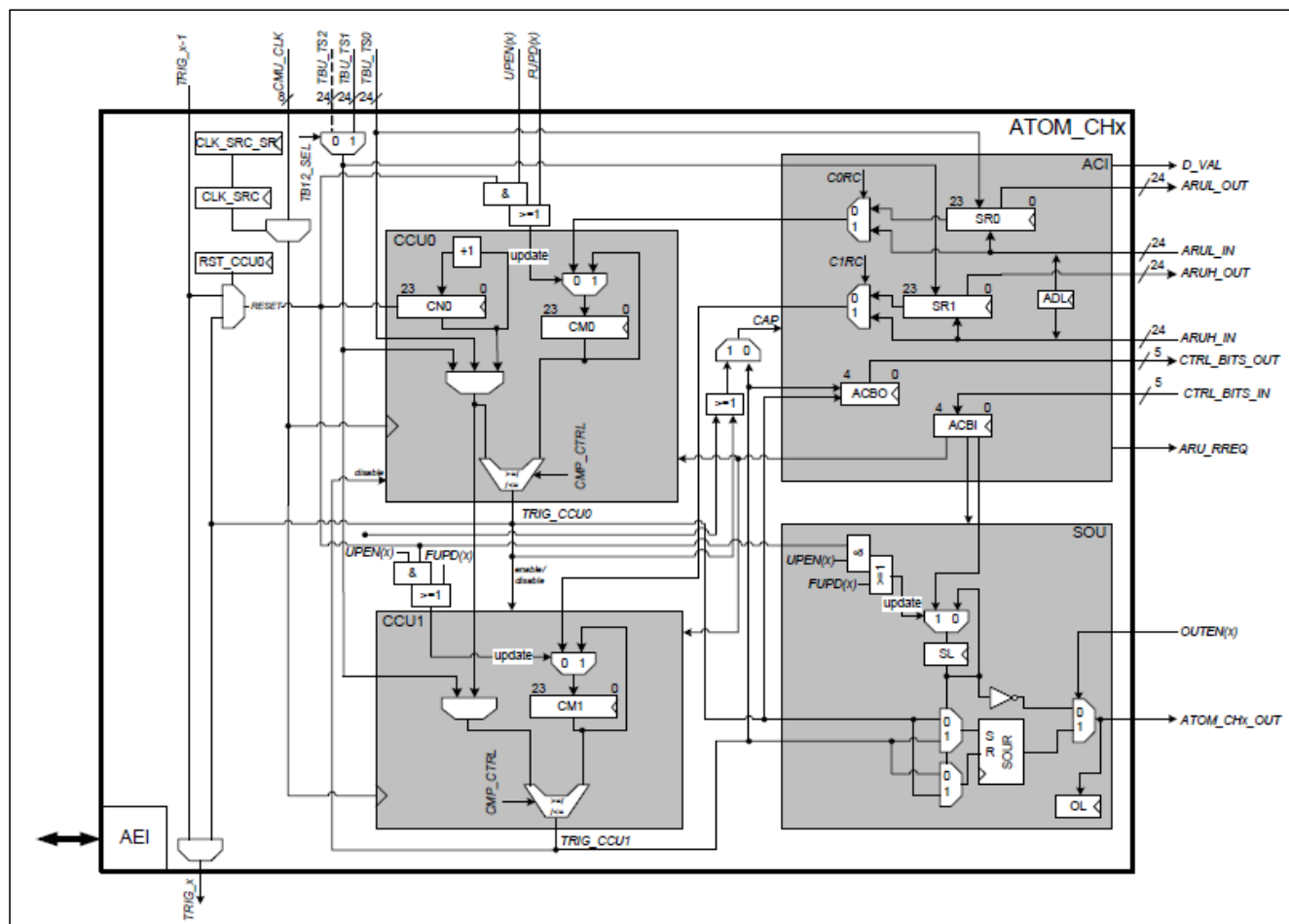
图5 ATOM通道结构
