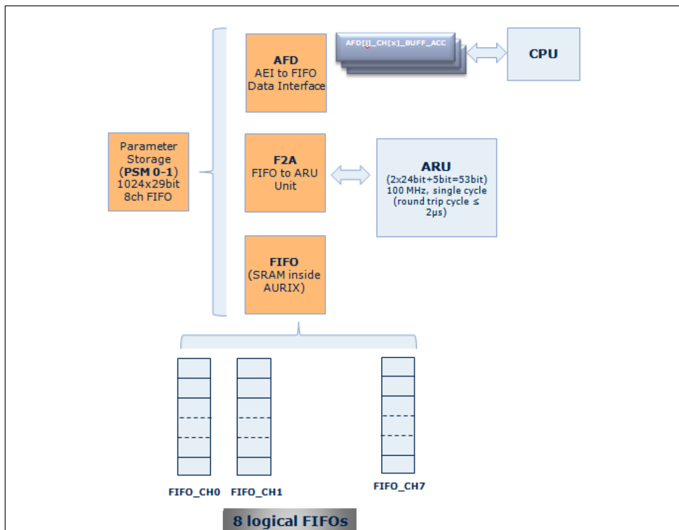
图19 PSM框图
