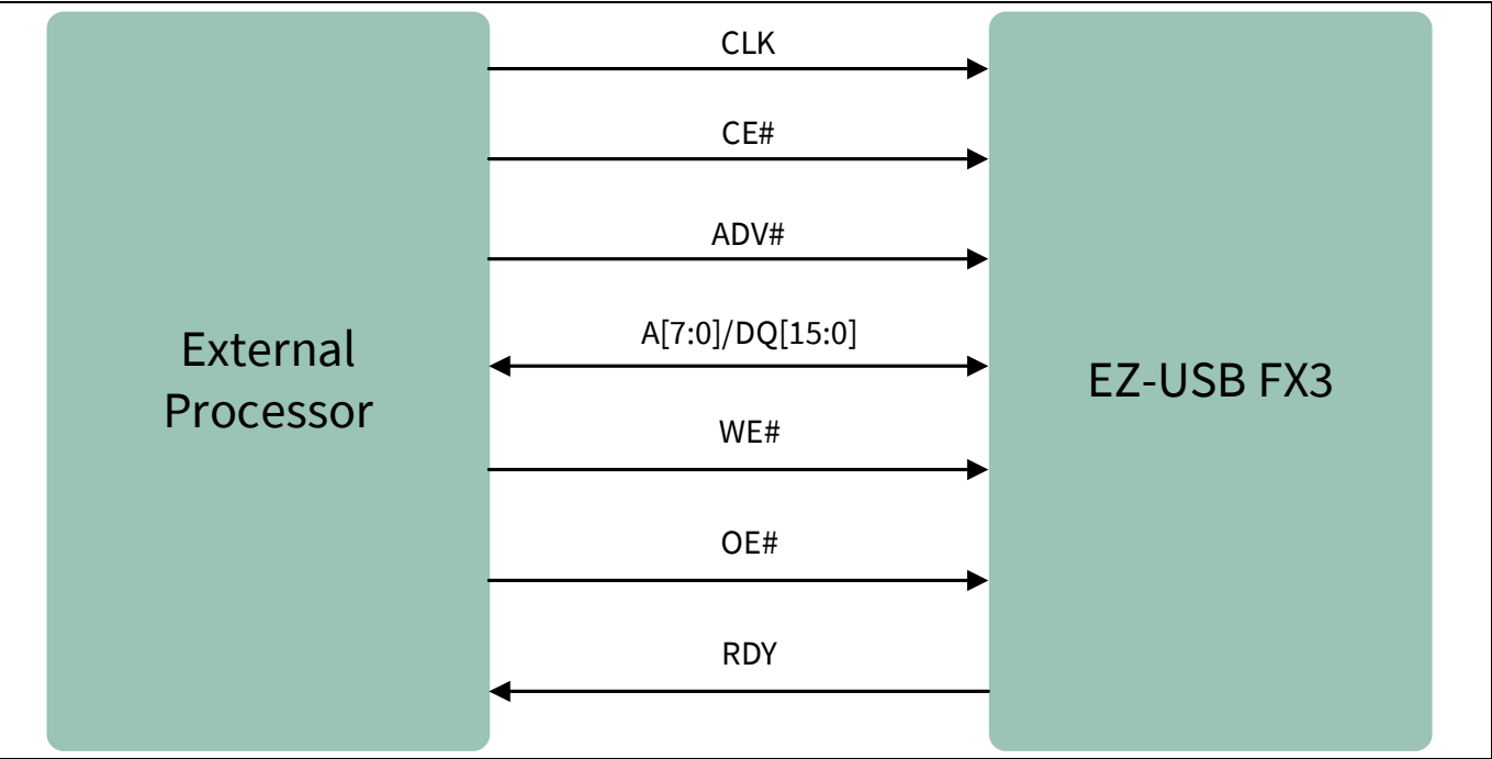
Figure 8 同步 ADMUX 接口
