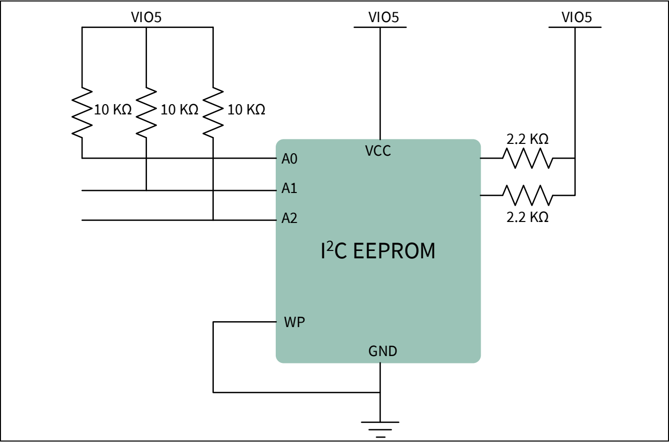
Figure 4 典型 I 2 C EEPROM 的引脚连接
