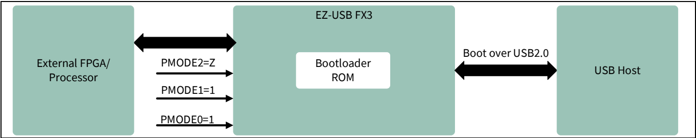
Figure 2 FX3 系统框图
