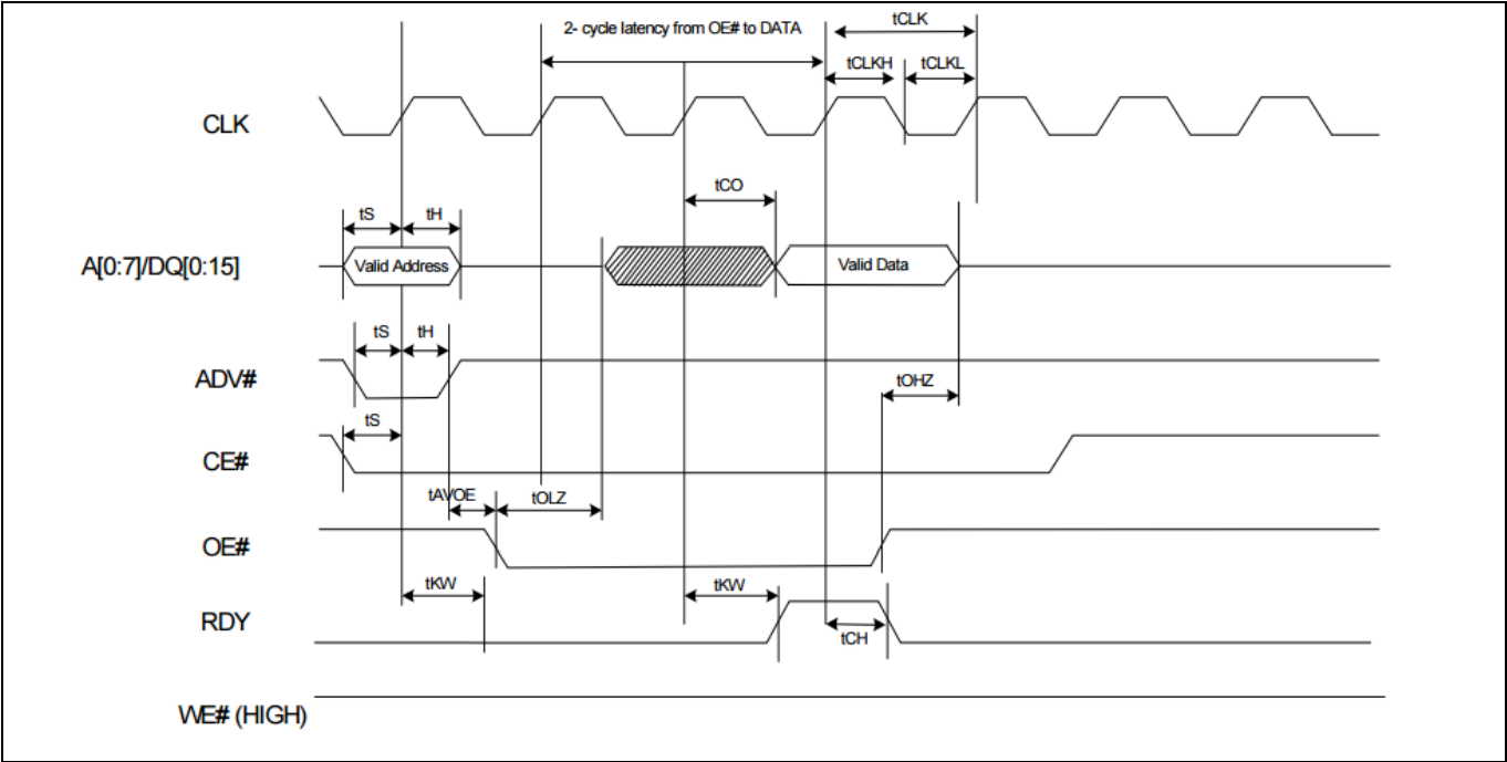
Figure 9 同步 ADMux 接口 — 读周期时序
