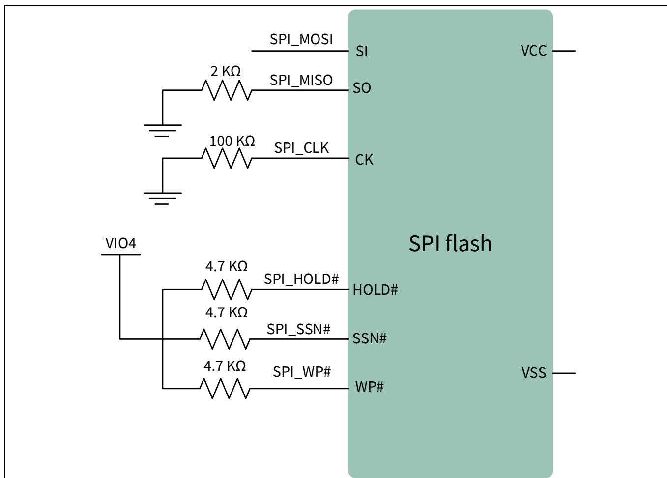
Figure 6 M25P40-VMN6TPB SPI 闪存的引脚连接示例
