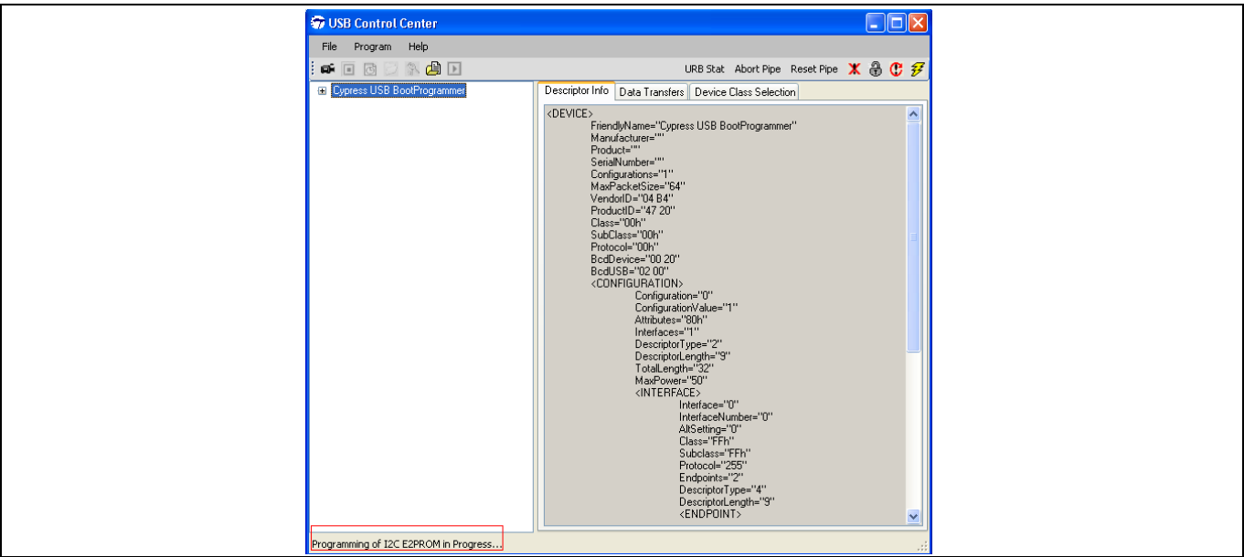
Figure 26 I 2 C EEPROM 在 Control Center 中的编程更新
