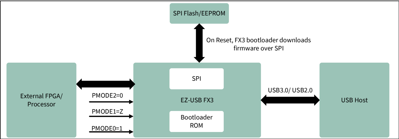
Figure 5 SPI 启动的系统框图
