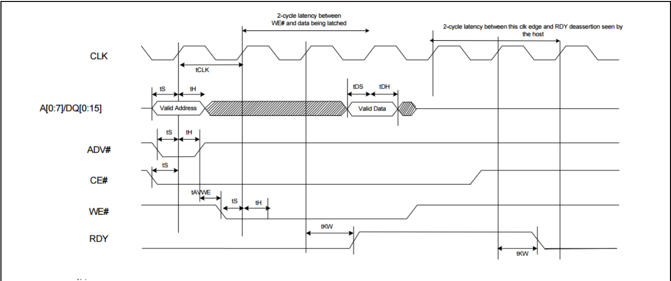
Figure 10 同步 ADMux 接口 — 写周期时序
