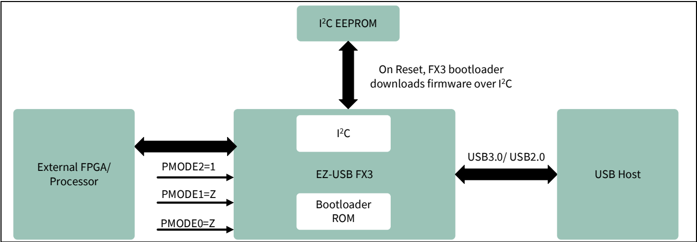
Figure 3 FX3 通过 I 2 C 启动的系统框图
