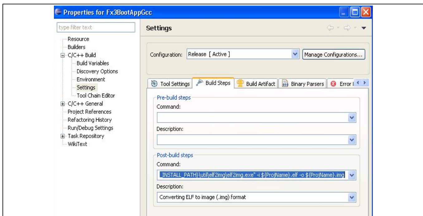
Figure 11 Eclipse IDE 中的编译后命令
