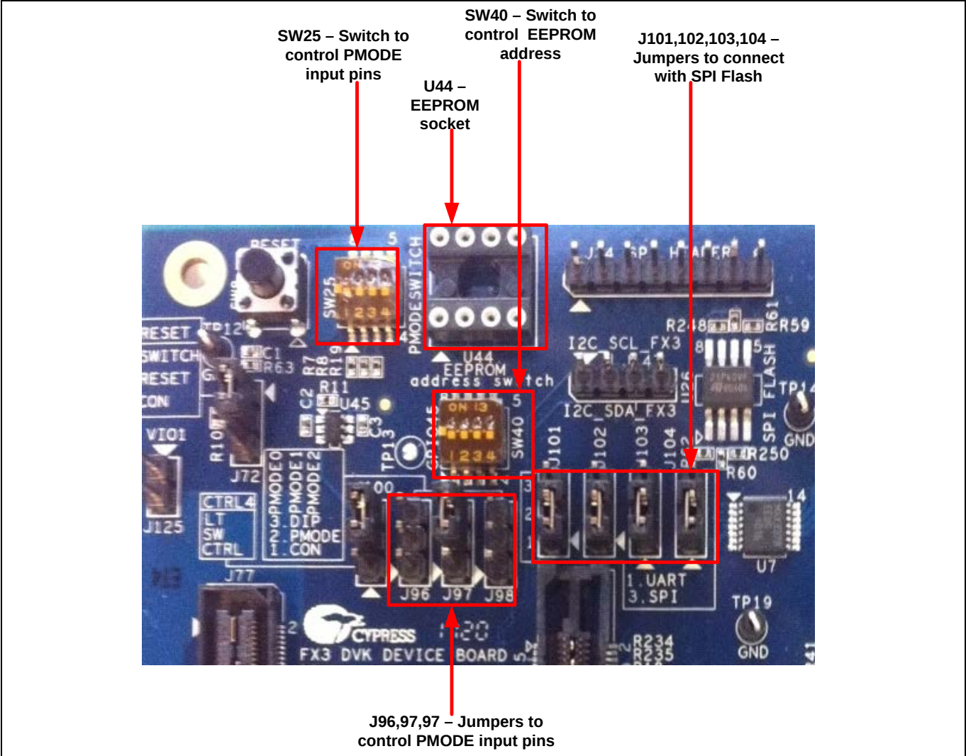
Figure 12 FX3 DVK 电路板: 用于启动的关键开关和跳线器配置
