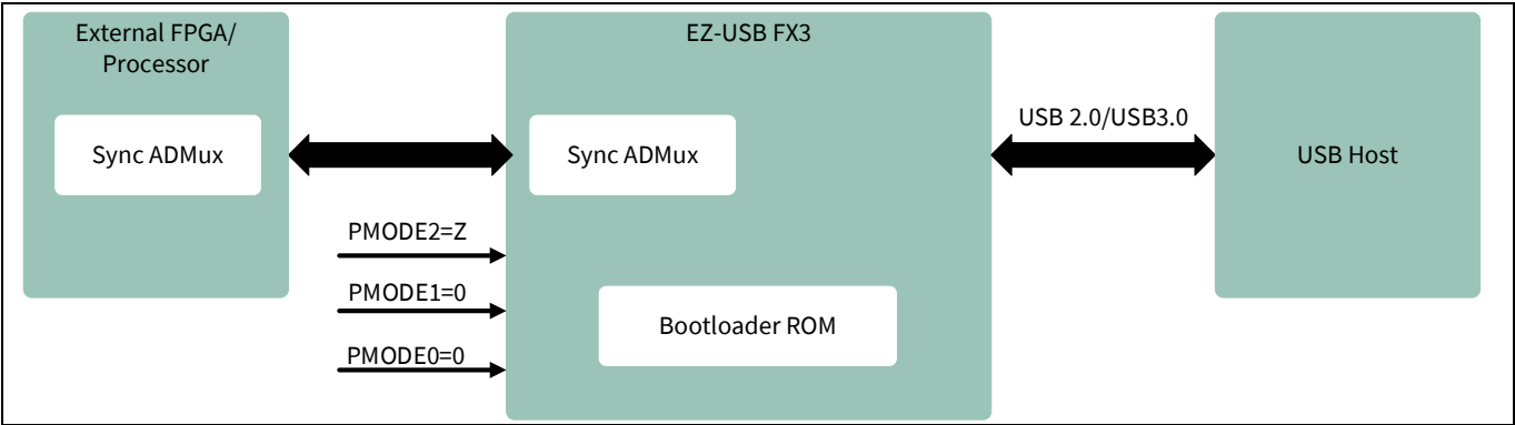
Figure 7 同步 ADMux 启动的系统框图
