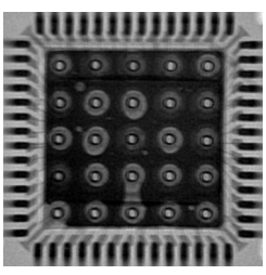
图 42. 装配的 X 射线图像
