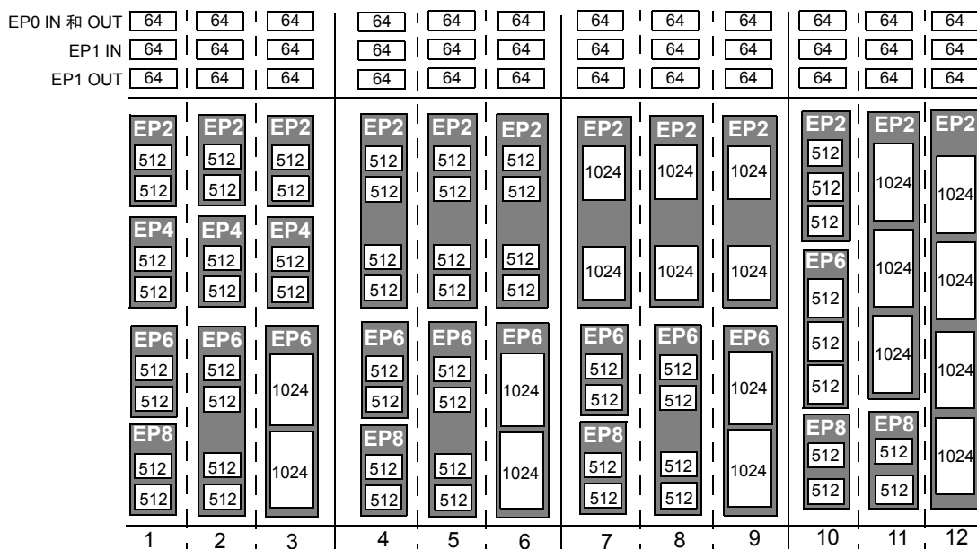
图 5. 端点配置
