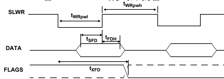
图 21. Slave FIFO 异步写入时序图 [20]
