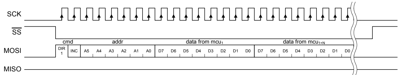
图 8. SPI 递增突发写入序列
