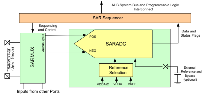
图 5. SAR ADC
