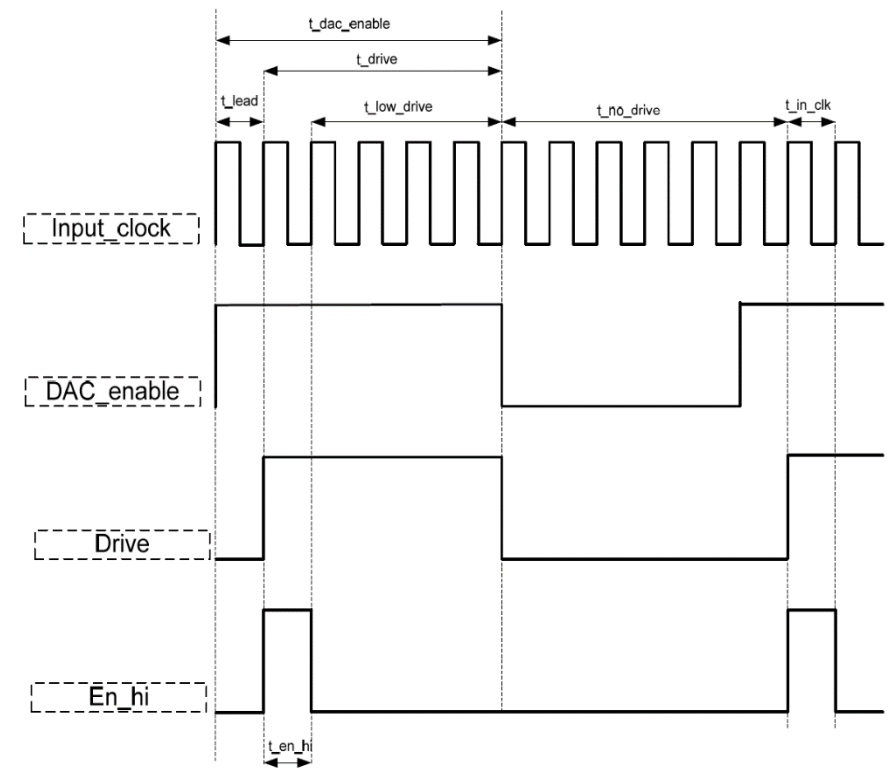
图 5. 控制信号时序图示例
