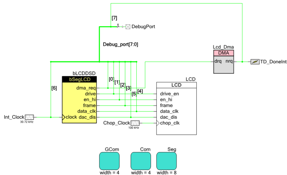
图 6 说明段显示器组件的内部原理图。该组件由以下器件组成：基本的段显示器组件、LCD 控制模块(LCD)组件、DMA 组件、2 个 LCD 端口，1 个数字端口、ISR 组件和 2 个时钟。
