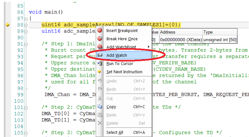
图 26. 查看变量
