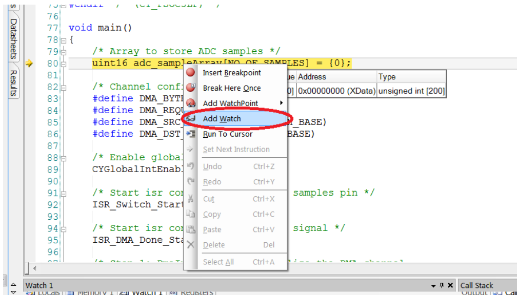
图 21. 查看变量
