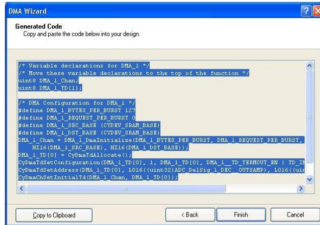
图 18. 生成代码
