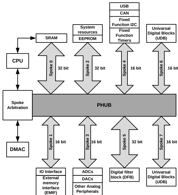
图 1. 外设集线器
