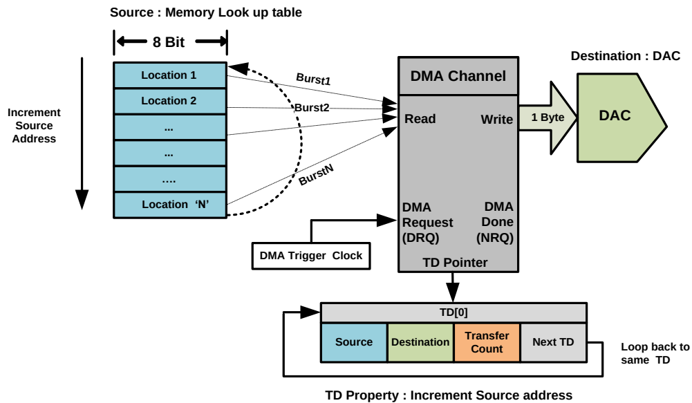
图 10. 存储器至外设传输的框图
