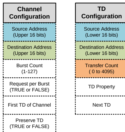
图 3. DMA 配置
