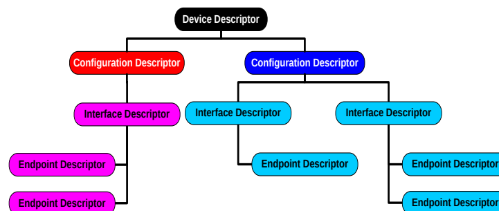
图 42. 带有两种配置的 USB 描述符
