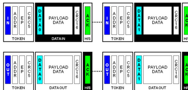
图 28. 数据切换示例
