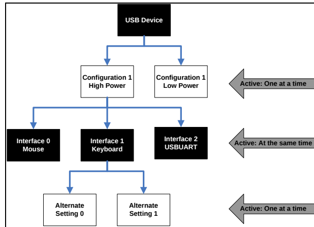
图 47. 配置框图
