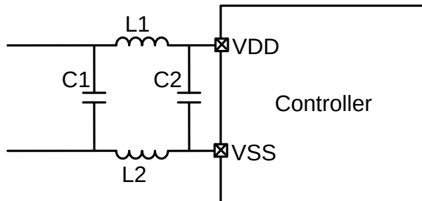
图 15. 控制器的供电引脚附近的滤波器
