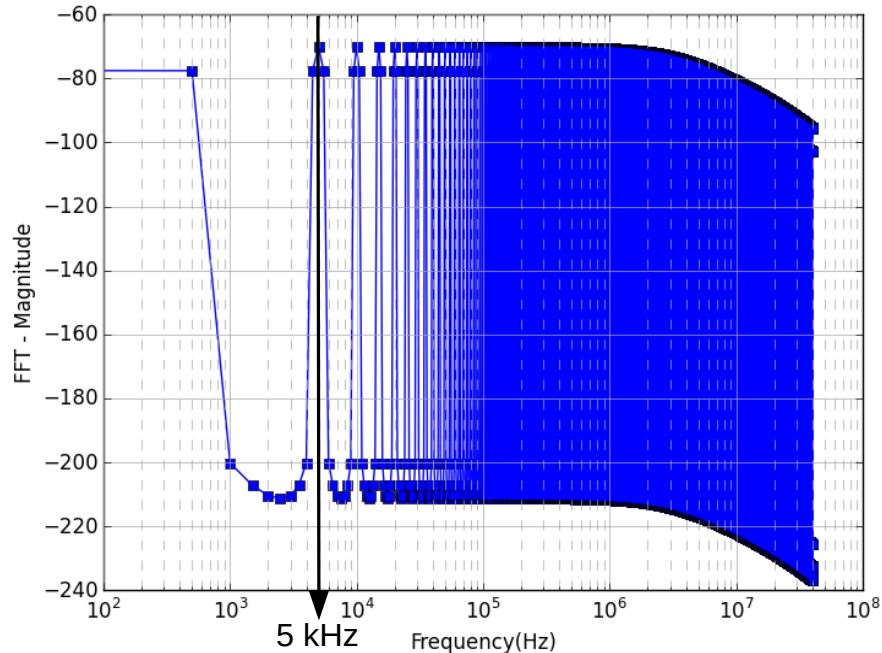
图 3. EFT – 5 kHz 突发：频谱
