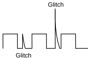
图 6. I/O 信号上的毛刺（由瞬变导致）
