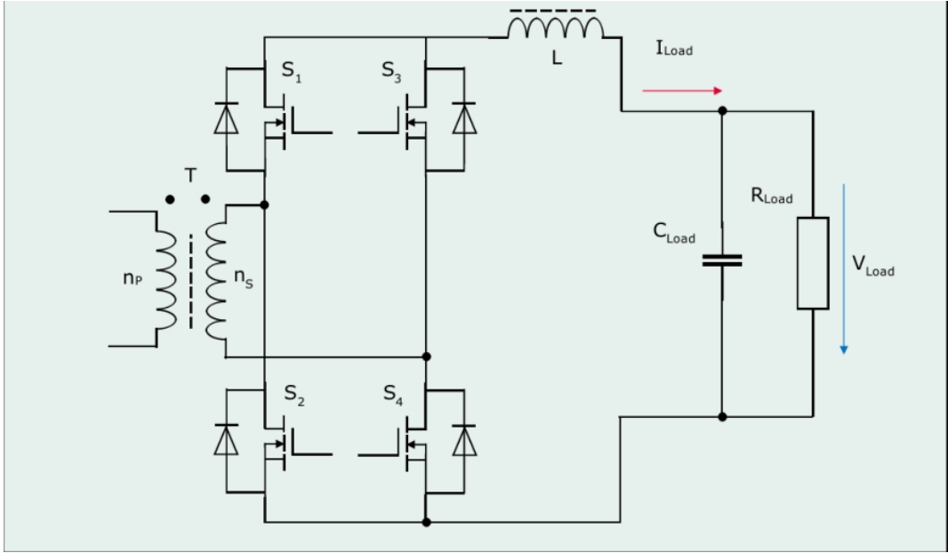
› Bidge rectifier
